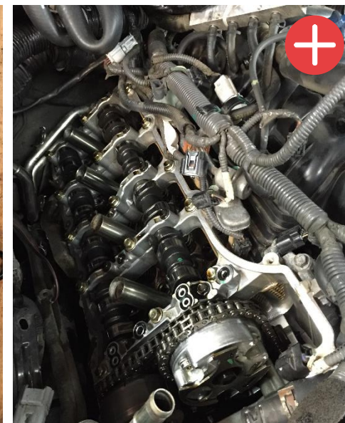
Вид двигателя Toyota Sequoia в момент съема клапанной крышки (пробег 300 000 км )
